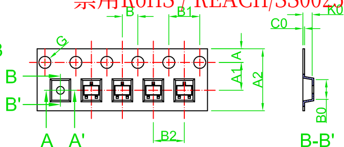
SOT-323
